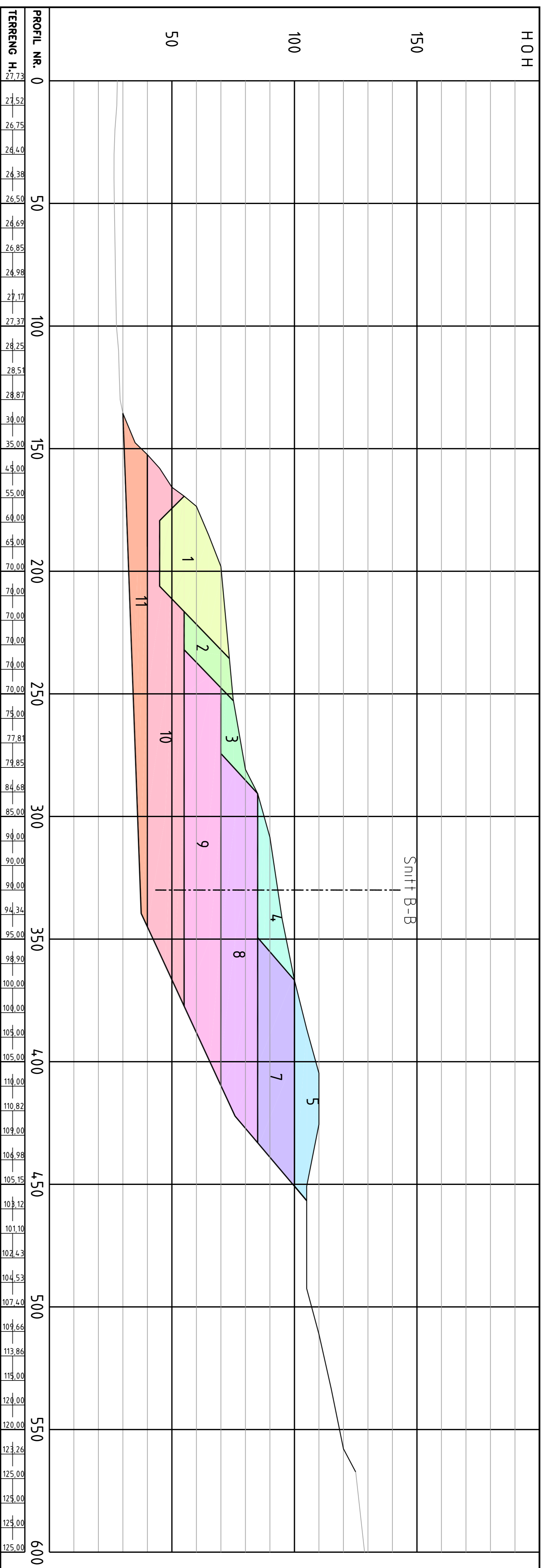
Snitt A-A
