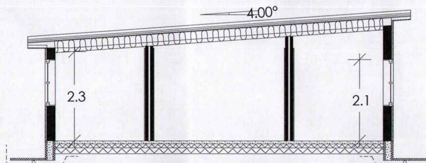
SNITT A-A
