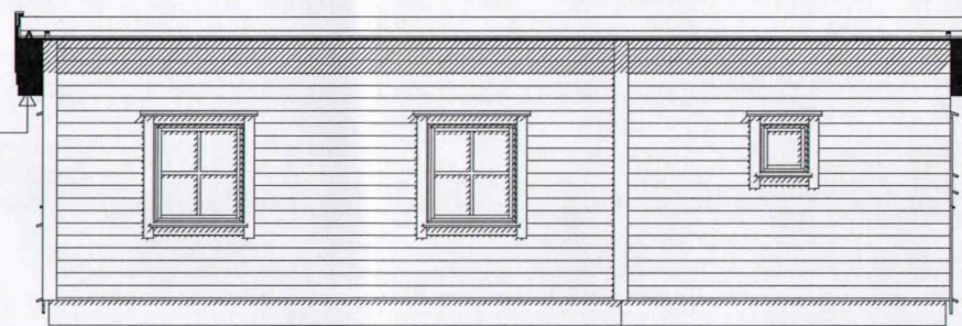
FASADE 3
