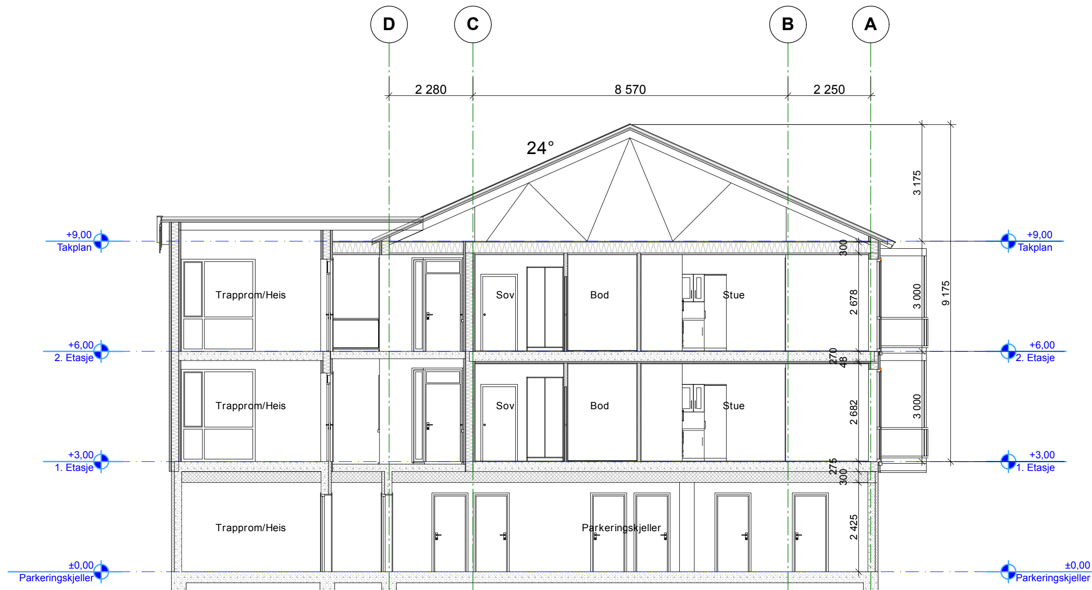
1:100 Snitt A
